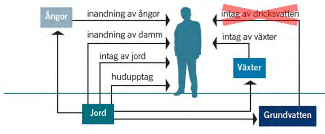
Figur 9 Exponeringsvägar som beaktas i beräkningen för PSRV jämfört med NV:s generella riktvärdesmodellen för hälsorisker 17
